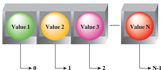
شکل ۱۲- آرایه اندیس‌دار
