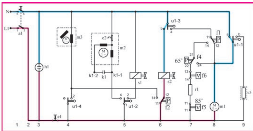
ت - نقشه تفکیکی مدار الکتریکی ماشین ظرفشویی اتوماتیک با الکتروپمپ دو جهت در مقطع زمانی ۲
