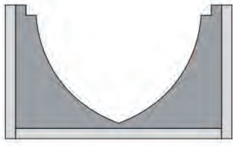
شکل ۴-۸۹ قالب یک بالشتک استاندارد
