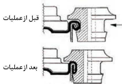
شکل ۸- نحوه عملکرد قرقره های ثانویه
