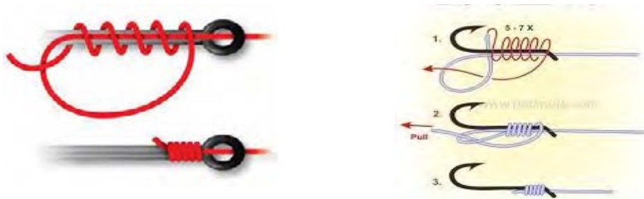
شکل ۲۴- دو نمونه گره برای بستن نخ مونوفیل‌مانت به قلاب ماهیگیری
