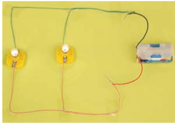
مدار موازی
