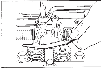
سوپاپ ها را فیلر گذاری کنید.
