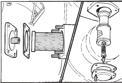
صافی بپمپ کمکی و پمپ روغن هیدرولیکی تراکتور را تمیز کنید.
