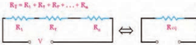
شکل ۳-۲- مدار سری با n مقاومت
