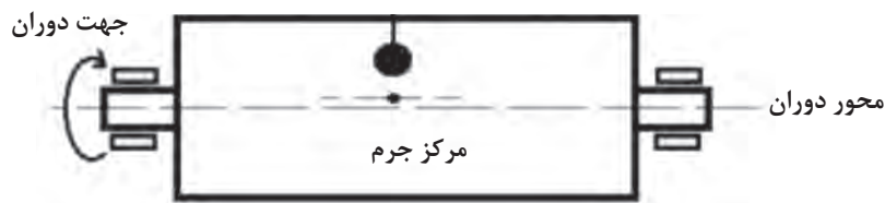
شکل ۵°- شماتیک بالانس استاتیک
