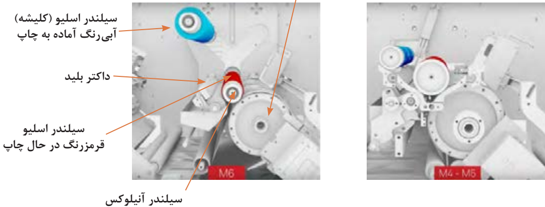
سیلندر فشار
