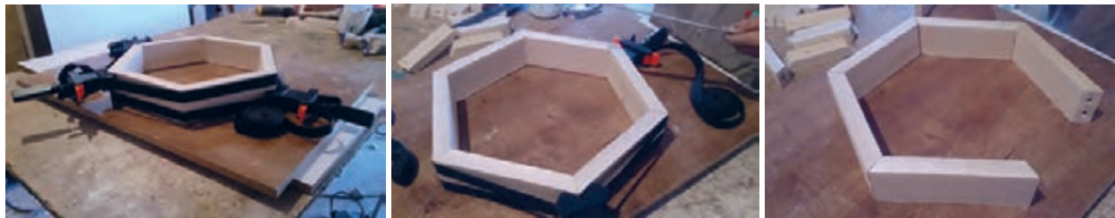
شکل ۳۷- جا زدن قیدها و بستن با گیره تسمه‌ای
