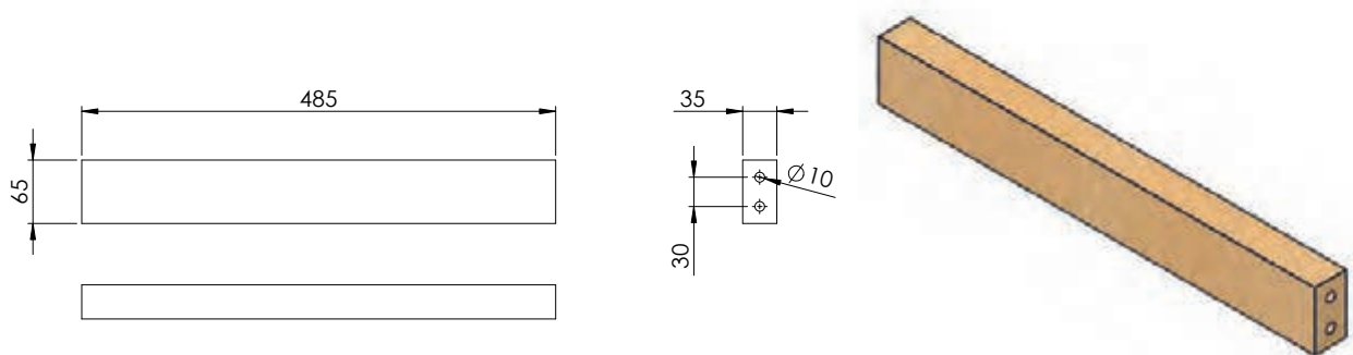
شکل ۶۹- نقشه فنی وادار کفی مبیل دو نفره
