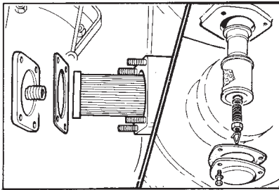
صافی بلمپ کمکی و پمپ روغن هیدرولیکی تراکتور را تمیز کنید.
