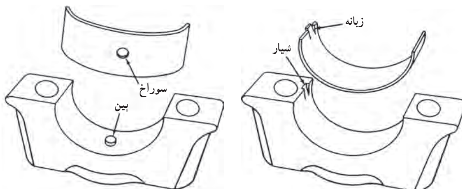
ب) یاتاقان زباندار
