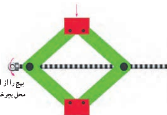
شکل ۳-۳- کاربرد پیچ در جک برای افزایش نیرو
