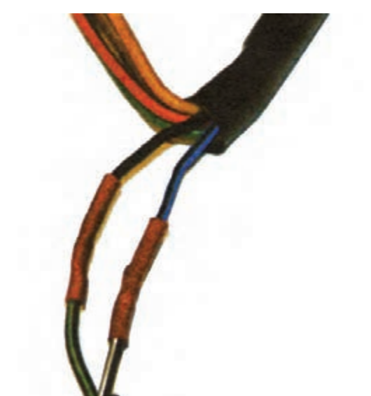
شکل ۶۵-۶- قرار دادن تیوب عایق روی محل اتصال سیم‌ها
