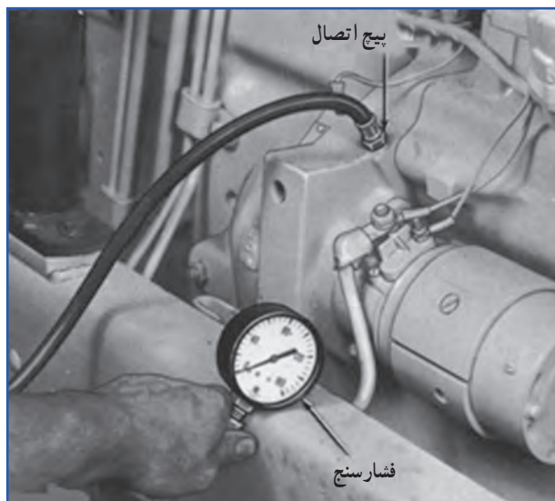
شکل ۱۳-۷- طرز اندازه‌گیری فشار روغن
