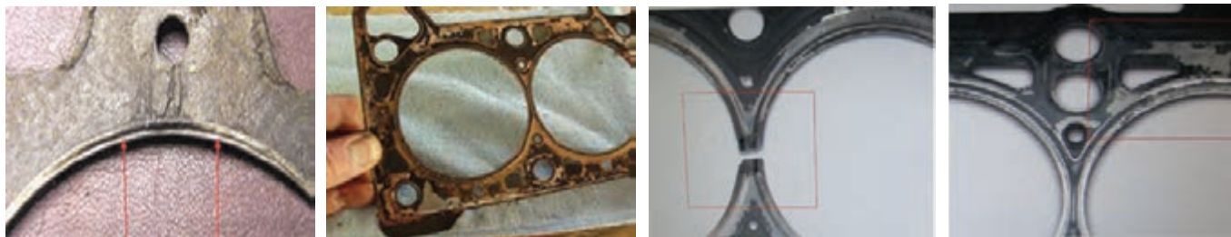
شکل ۵۰-۴- نواحی سوخته شده واشر سیلندر
