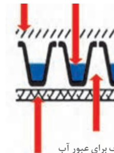
شکاف برای عبور آب باران اضافی و گردش هوا لایه تشک حفاظتی
