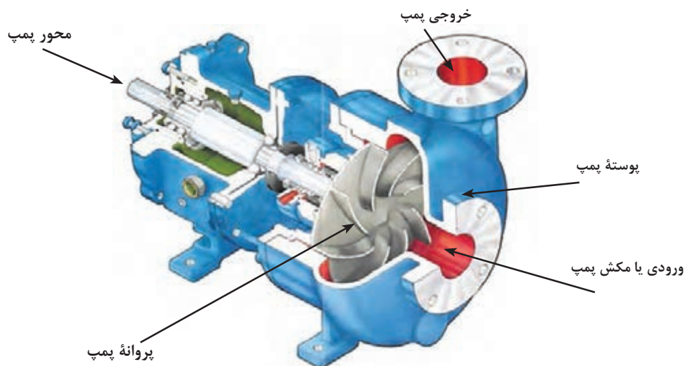
شکل ۴- نمایی از ساختمان پمپ گریز از مرکز با یک نوع پروانه متفاوت
