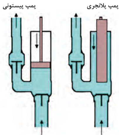
شکل ۱۶- تفاوت پمپ پیستونی و پلانجری
