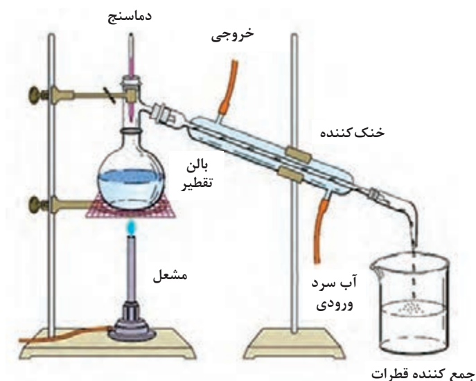
شکل ۶- سامانه تقطیر ساده
