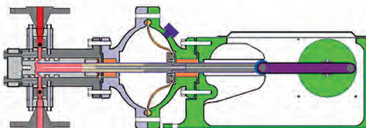
شکل ۱۵- پمپ پلانجری
