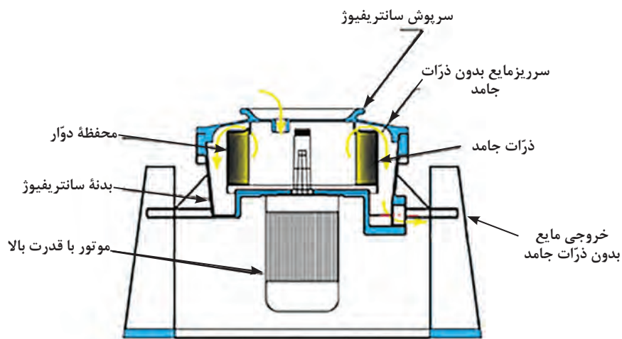
شکل ۳۸- اجزای یک نمونه سانتریفیوژ صنعتی
