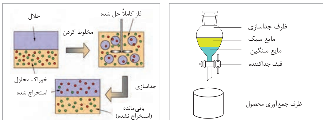
شکل ۱۱- فرایند استخراج مایع - مایع
