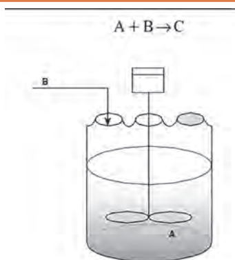
شکل ۱۱- راکتور نیمه پیوسته
