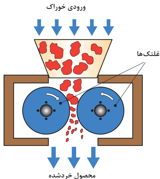
شکل ۴۴- خردکن غلتکی
