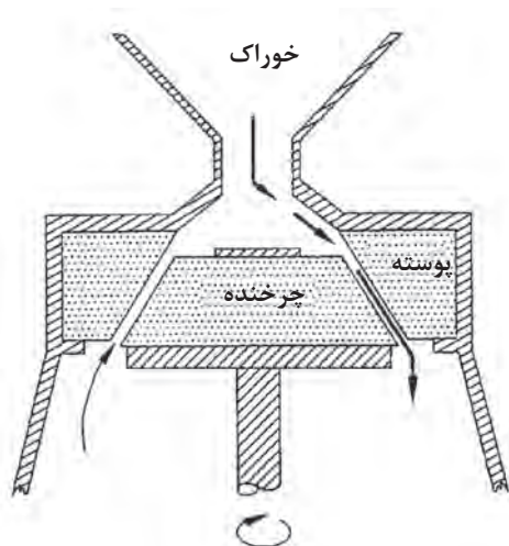
شکل ۴۷- طرح ساده‌ای از آسیاب کلوییدی
