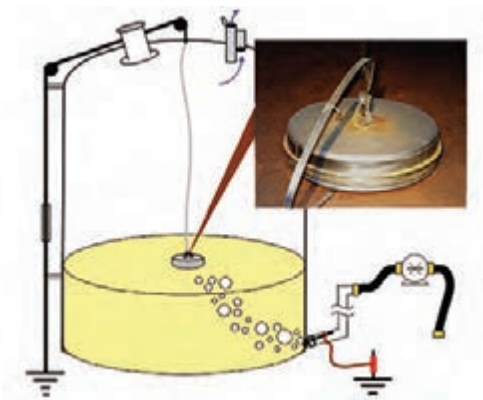
شکل ۲۵- تخلیه الکتریسیته ساکن مخزن به زمین
