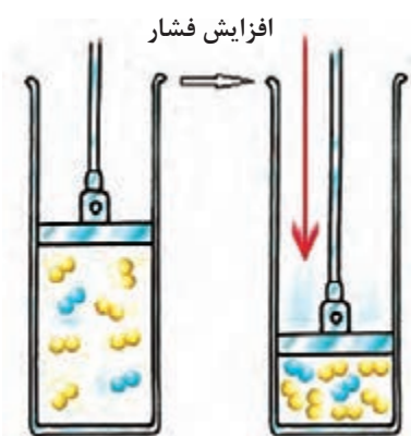
شکل ۱- تأثیر فشار بر سرعت واکنش
