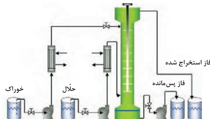
شکل ۱۵- فرایند استخراج مایع - مایع با تماس‌دهنده‌های ستونی
