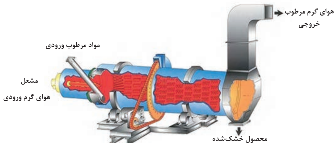
شکل ۱۳ - عملکرد خشک‌کن
