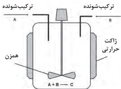
شکل ۱۲- راکتور نیمه پیوسته
