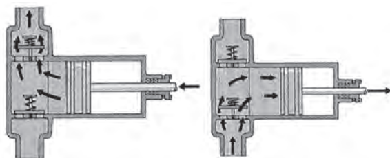
شکل ۱۴- شیوه عملکرد پمپ پیستونی
