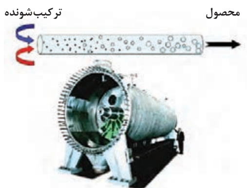
شکل ۸- راکتور لوله‌ای
