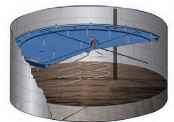
شکل ۱۸- مخازن سقف شناور بیرونی
