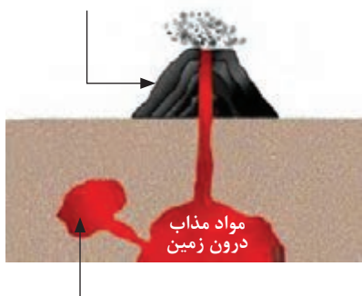
شکل ۳- سنگ آذرین که درون زمین ایجاد می‌شود
