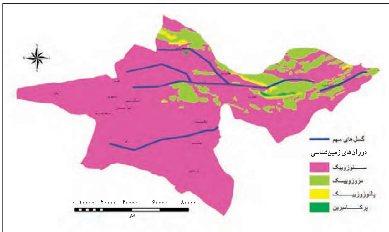
شکل ۲۵-۱ گسل‌های تهران
