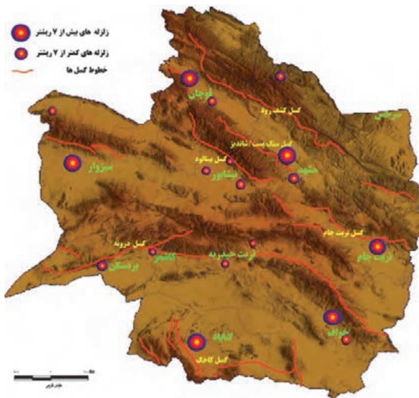
شکل ۱۳-۱ نقشه پراکنده‌گی گسل‌های استان خراسان رضوی
