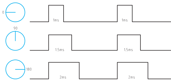
تصویر ۲۹- پالسیهای فرمان سروو موتور
