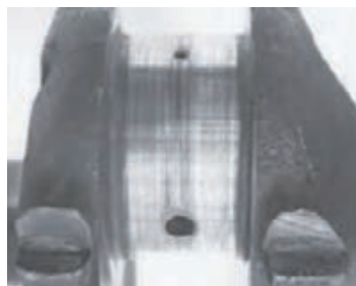
ایجاد خراش روی میل لنگ
