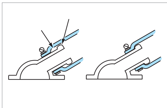
شکل ۲۴- برخی نکات مهم بررسی، عیب‌یابی و بستن مدار خنک‌کاری
