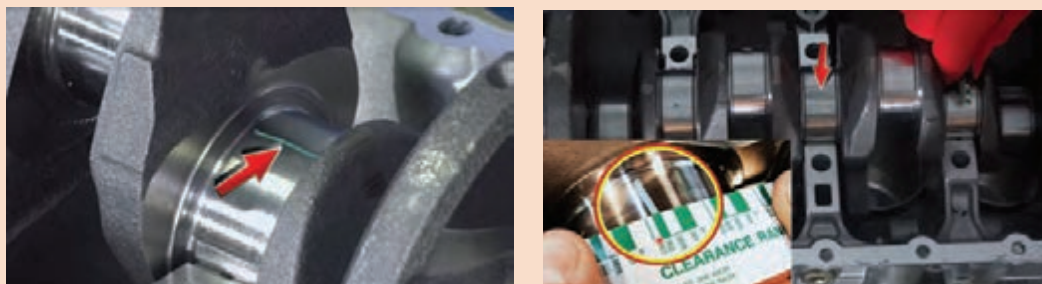
شکل ۹۷- برخی از نکات استفاده از پلاستی گیج برای تشخیص فاصله بین میل‌لنگ و یاتاقان ثابت
