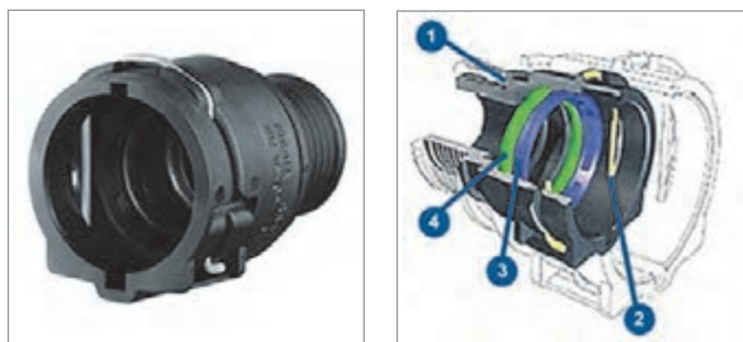
شکل ۱۶- رابط اتصال سریع در شیلنگ‌ها (الف) (ب)
