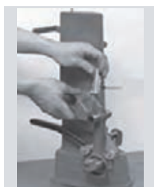
بررسی خمیدگی شاتون
