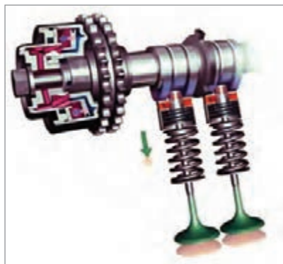
شکل ۳۹- سیستم VVT
