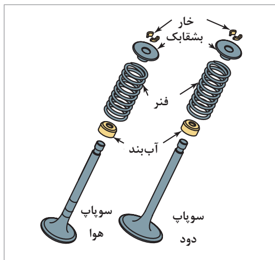
شکل ۸۳- اجزای سوپاپ‌ها
