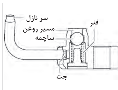
شکل ۱۱- جت روغن
