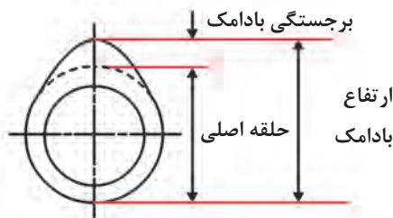
(الف) ارتفاع بادامک
