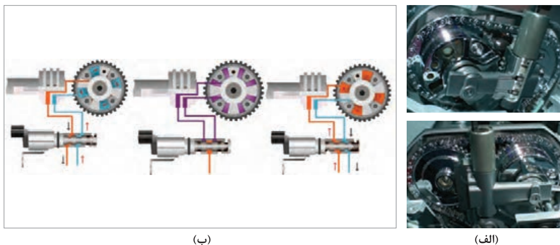
شکل ۴۳- موقعیت شیر برقی VVT و عملکرد آن
