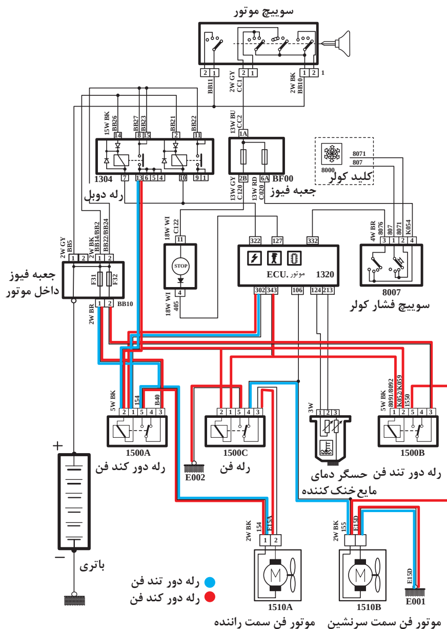
شکل ۴۵- عملکرد مدار فن - دوفن، دو دور
