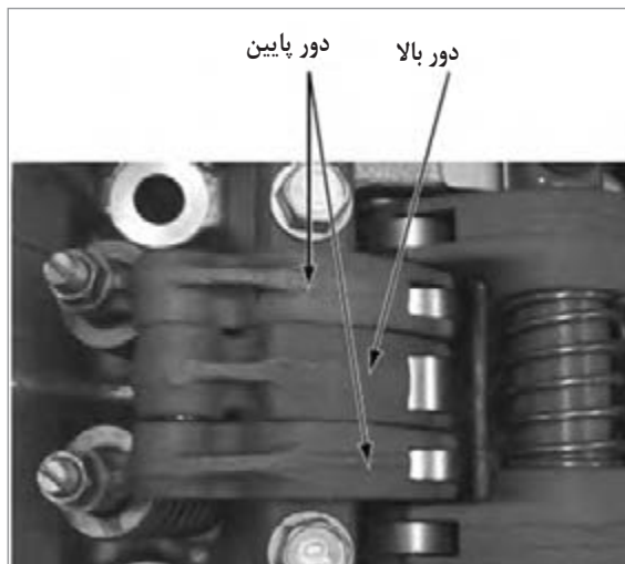
الف) مجموعه اسبک غلتکی محرک دو سرعته (ارتفاع متغیر) (موتور OHV - OHC)
