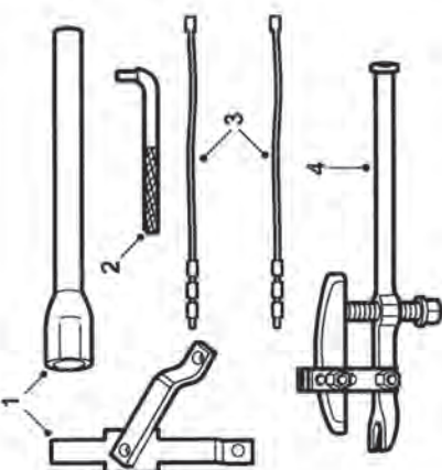
شکل (۱-۴۰) ابزار باز کردن محور چرخ جلو
