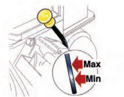
شکل (۲-۶۱) حداکثر و حداقل گیج روغن
