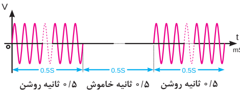
شکل ۸۳ - مشخصات سیگنال اشغال خط
