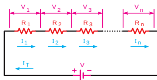
شکل ۱۴ - مقادیر ولتاژ در مدار سری
