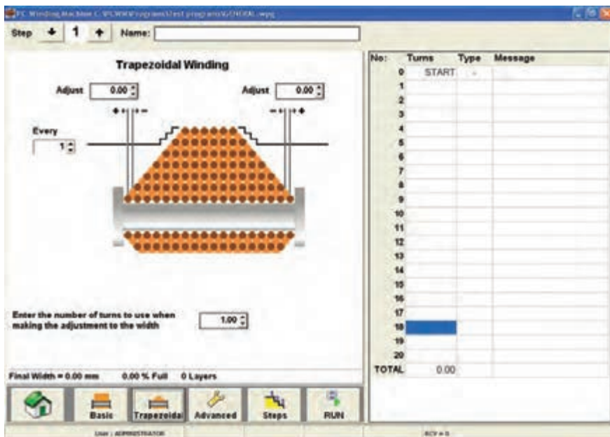
شکل ۳۲- نمونه دیگری از منوی دستگاه بوبین پیچ
