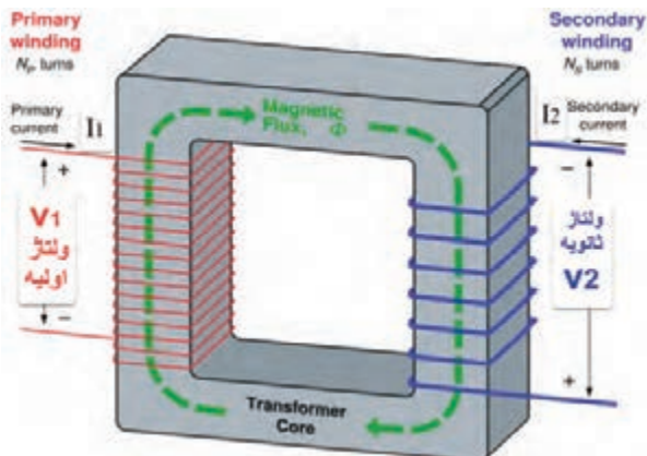
شکل ۲۲- رفتار ترانسفورماتور
