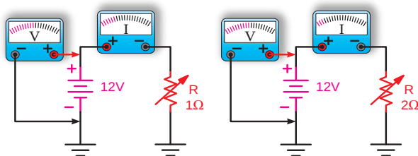
ب - رابطه جریان با مقدار مقاومت
