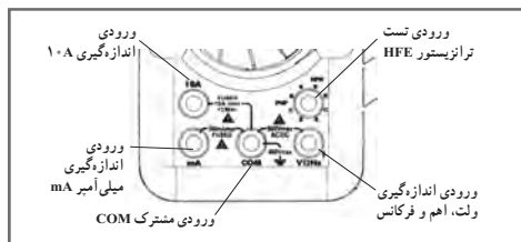
شکل ۲۷- ورودی‌های مولتی متر دیجیتالی
