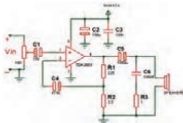
شکل ۷۸- مدار تقویت کننده با ولوم کنترل شدت صوت
