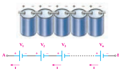
شکل ۱۸- اتصال سری پیل‌ها
