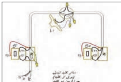
شکل ۱۵۲- مدار کلید تبدیل (برق از کلید) چراغ بین دو کلید
