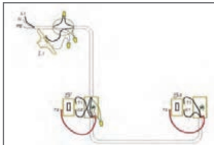
شکل ۱۵۱- مدار کلید تبدیل (برق از چراغ)
