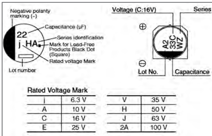
شکل ۱۰ - کدگذاری خازن های الکترولیتی
