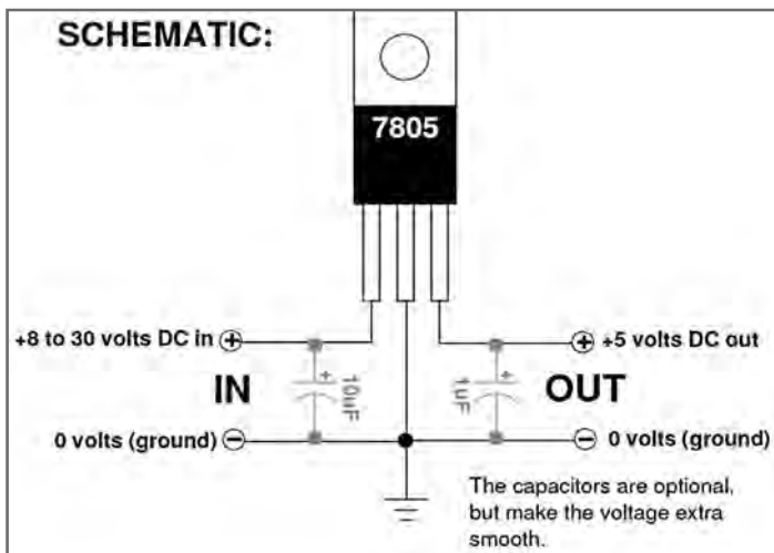
شکل ۱۱ - یک نمونه از برگه اطلاعات آی سی رگولاتور
