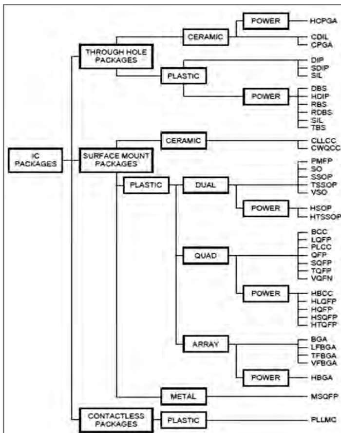
شکل ۱۵ - نمودار انواع بسته‌بندی‌های SMD
