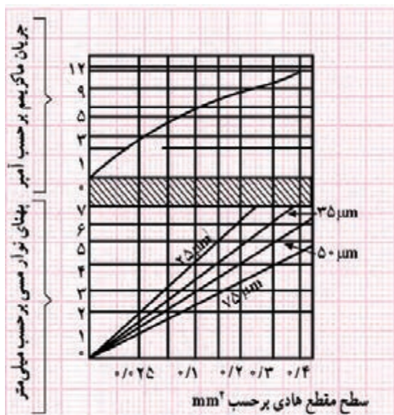
شکل ۱۲۳- محاسبات فیبر مدار چاپی
