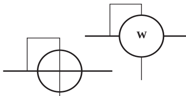
شکل ۷۷ - علامت‌های فنی وات‌متر
