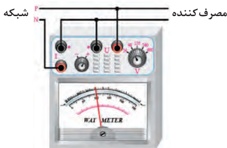
شکل ۷۸ - نحوه اتصال وات‌متر به شبکه برق شهر و مصرف‌کننده
