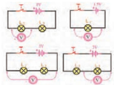
شکل ۱۲ - اتصال ولت متر به مدار سری
