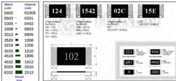
شکل ۷- نمونه دیگری از رمز «عدد-حرف»
