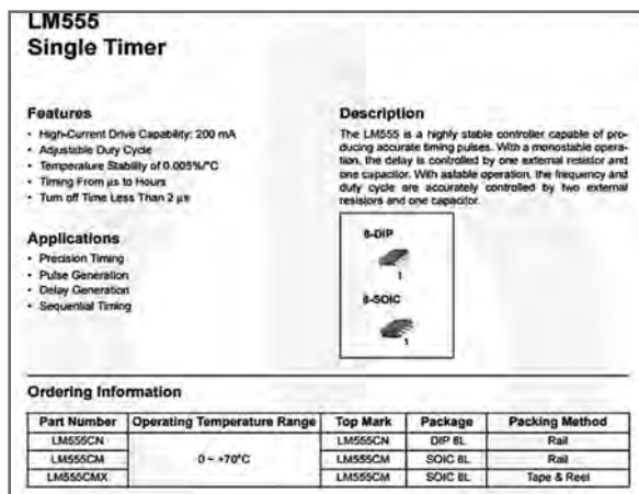
شکل ۱۲ - یک نمونه برگه اطلاعات تایمر LM555
