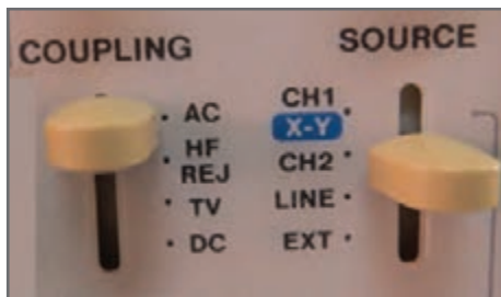
شکل ۶۹- وضعیت‌های کلید Source
