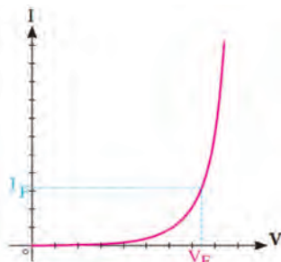
شکل ۴۱- نمایش مقاومت استاتیکی
