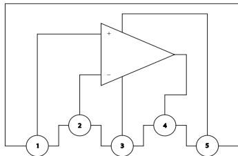
شکل ۷۷- بلوک دیاگرام TDA۲۰۰۳
