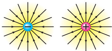
شکل ۵ - جهت خطوط نیرو
