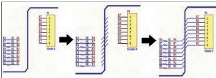
شکل ۲۶- روش کشیدن باس و اتصال باس انتری
