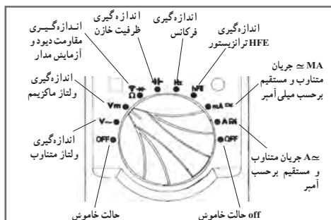
شکل ۲۶- سلکتور مولتی متر دیجیتالی
