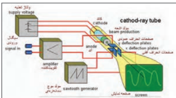
شکل ۴۸ - نمایی از قسمت های اسیلوسکوپ
