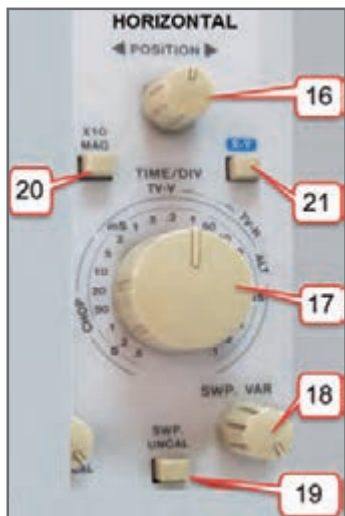
شکل ۶۴ - کلیدها و ولوم های بخش افقی
