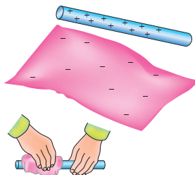
شکل ۲- پس از مالش دادن یک میله شیشه‌ای به پارچه ابریشمی، آنها دارای بار الکتریکی می‌شوند.
