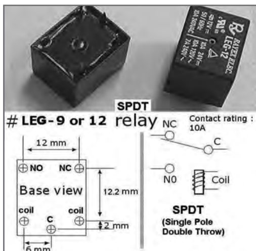
شکل ۴- مشخصات فنی یک نمونه رله
