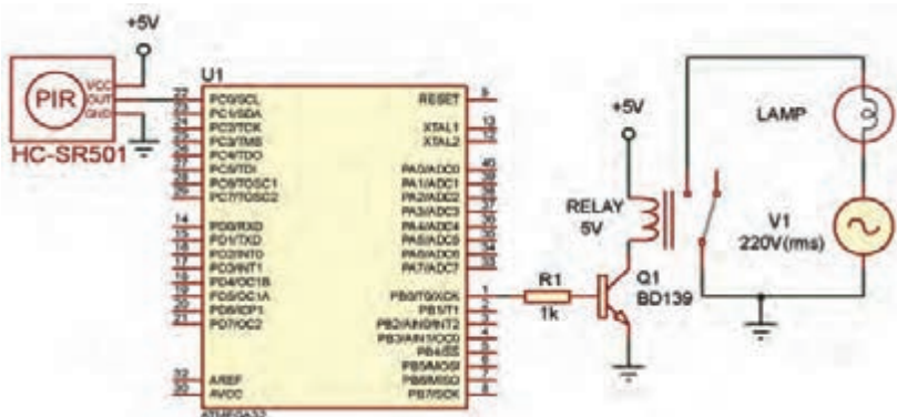
شکل ۸۳- نقشه الکترونیکی اتصال مازول HC-SR501 به میکروکنترلر
