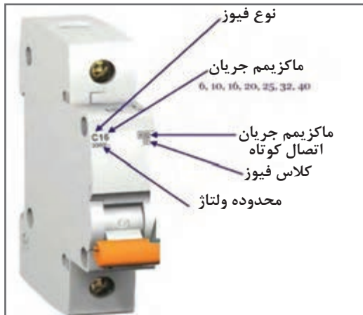
شکل ۱- مشخصات یک نوع فیوز مینیاتوری
