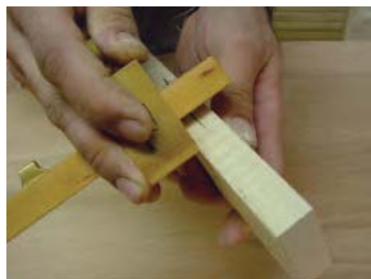
شکل ۹-۱۵- تعیین وسط نر چوب به وسیله‌ی فکاش تیره‌دار.
