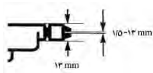
شکل ۱۹-۵۰- دهانه‌ی سه‌نظام تا قطر ۱۳ میلی‌متر.
