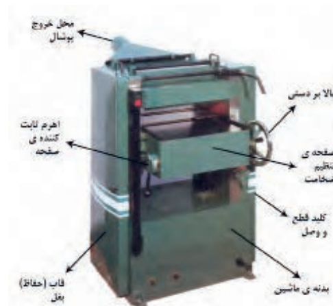
شکل ۷-۵- مشخصات ظاهری ماشین گندگی.
