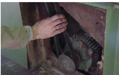
شکل ۶-۶ - کنترل شل و سفتی تسمه.
