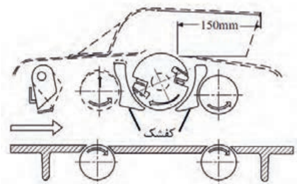
شکل ۷-۱۵ - کفشک‌ها.
