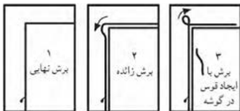
شکل ۳۶-۱۵. نمونه‌ی حرکت تیغه اره برای برش یک گنچ.
