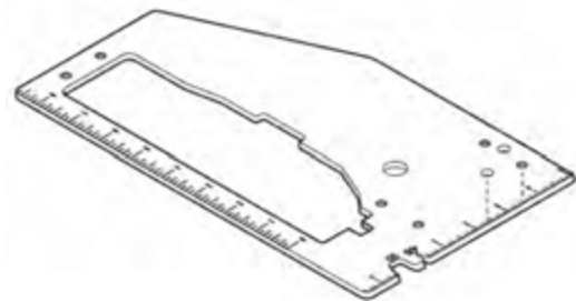
شکل ۲-۱۳- صفحه‌ی ماشین اره گرد دستی.
