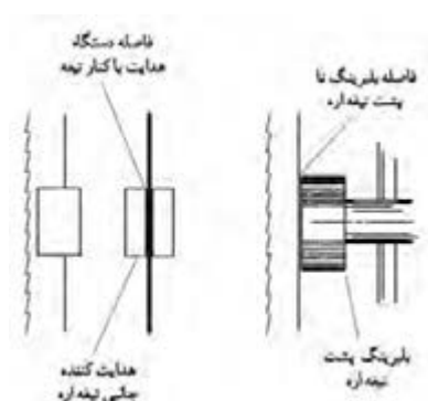
شکل ۹-۲- موقعیت دستگاه هدایت نسبت به تیغه اره.
