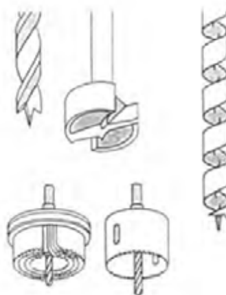
شکل ۱۹-۲۴- مته‌های مفصوص چوب.
