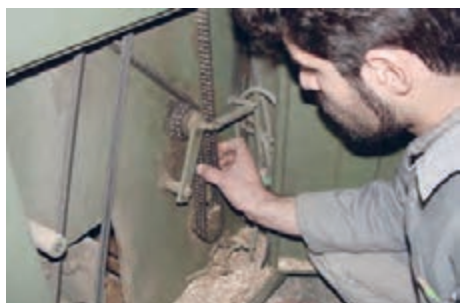
شکل ۲۷-۷. تنظیم و آزمایش سفتی زنجیر انتقال نیرو.
