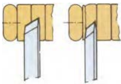
شکل ۱۱-۲۸. پی‌گونی کار با مغار مورب.
