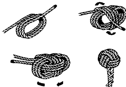
نحوه زدن گره پنجه میمونی
