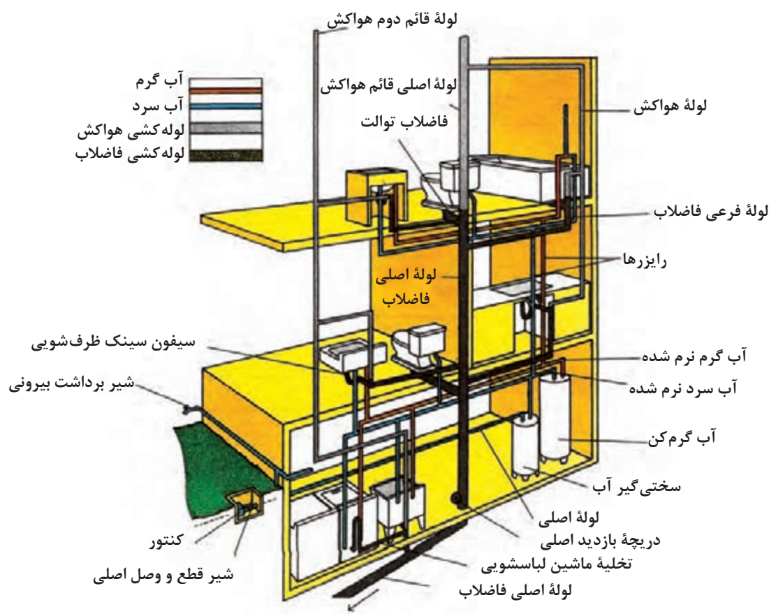
شکل ۴-۲- لوله‌کشی آب سرد و گرم مصرفی و فاضلاب ساختمان
