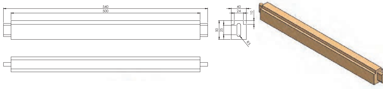
شکل ۶- نقشه فنی قید بالا
