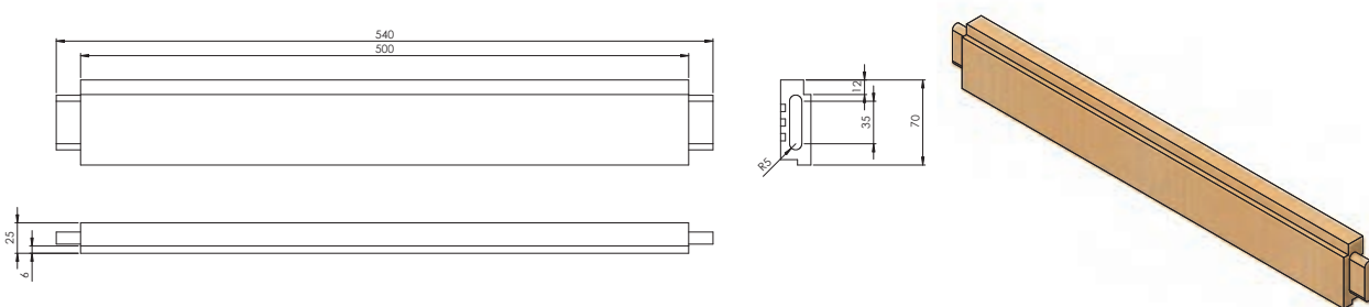
شکل ۷- نقشه فنی قید عقب
