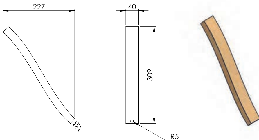
شکل ۷۰- نقشه فنی وادار پشتی
