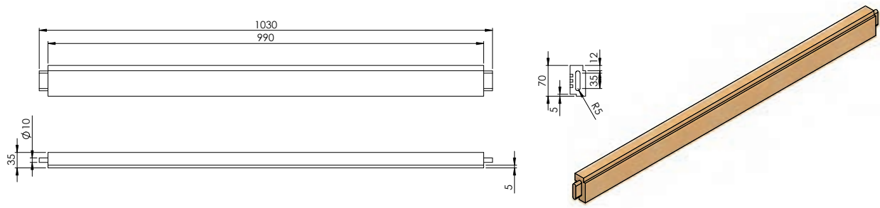
شکل ۶۷- نقشه فنی قید عقب
