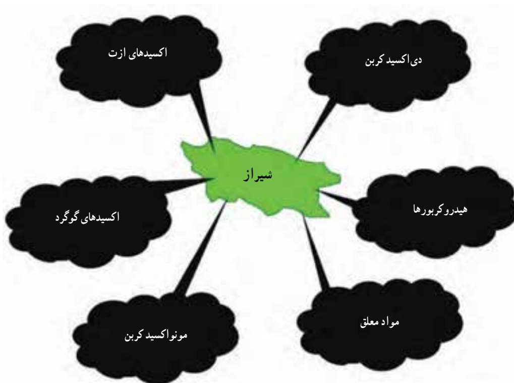
شکل ۴۵-۱- منابع آلوده‌کننده هوای شهر شیراز
