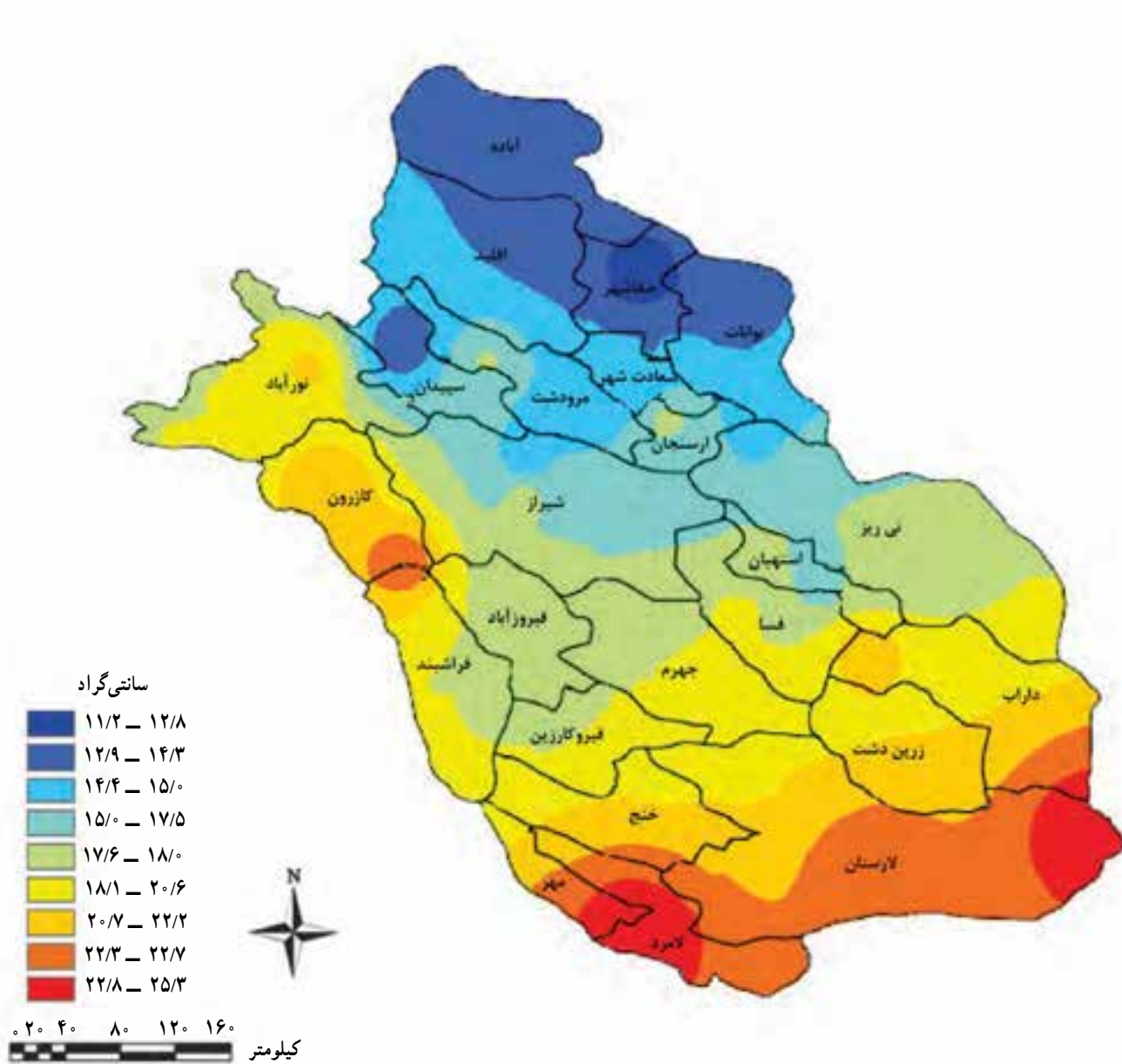
شکل ۱۴-۱- نقشه هم دمای استان فارس
