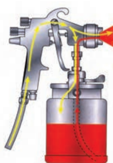
شکل ۱۸-۸- پیستوله کاسه پایین.
