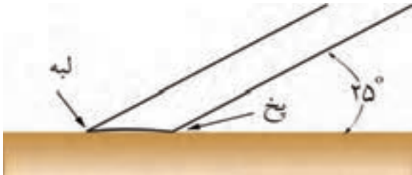
شکل ۳۲-۳- زاویه‌ی پیغ تیغ رنده‌ها باید ۲۵ درجه باشد.
