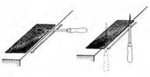
شکل ۳-۴۴- مصقل‌کشی لیس.
