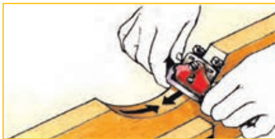
شکل ۳-۴۰- لیسسه کاری داخل قوس‌ها.
