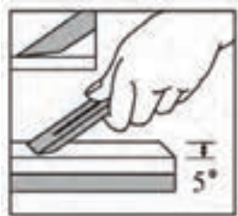
شکل ۱۴۹-۳- استقرار صمیغ تیغه رنده روی سنگ نفت.
