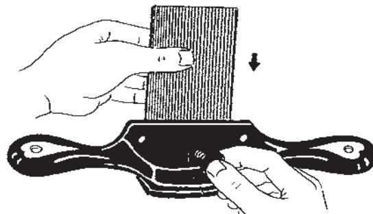
شکل ۳-۳۹- طریقه‌ی نصب لیسسه به رنده‌ی بال کبوتری.
