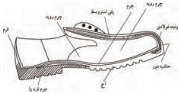
شکل ۹-۱- کفش ایمنی.
