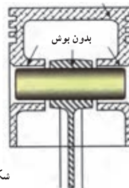
(الف) انگشتی شناور
