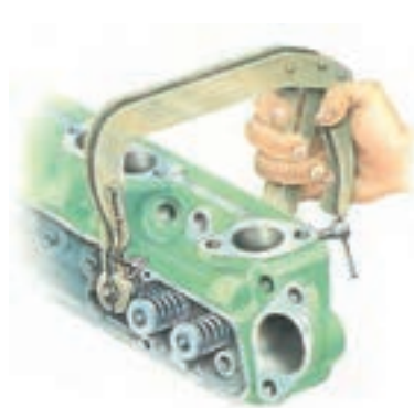
شکل ۴-۱۷- نحوه قرار دادن سوپاپ باز کن روی سوپاپ‌ها
