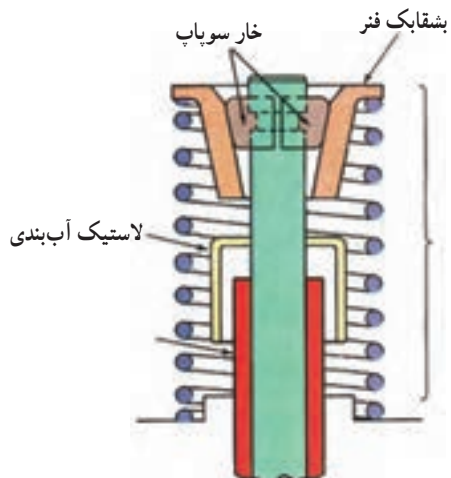
(ب) اجزای جمع شده سوپاپ
