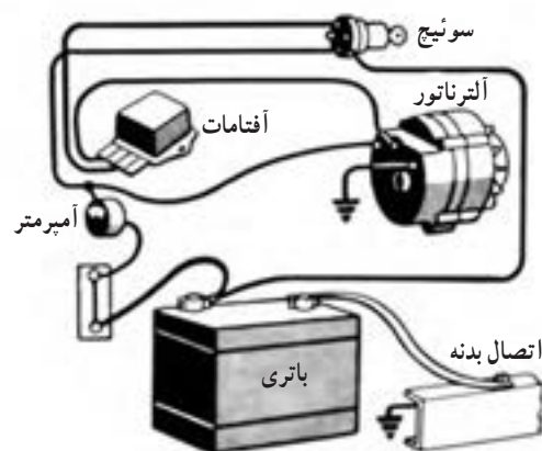
(الف) مدار شارژ آلترناتور
