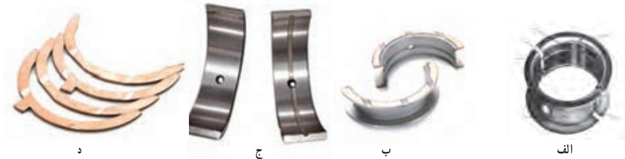
شکل ۳۷-۲ یاتاقان
