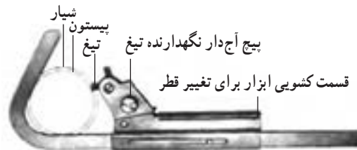
(الف) ابزار تمیزکننده شیار رینگ‌ها
