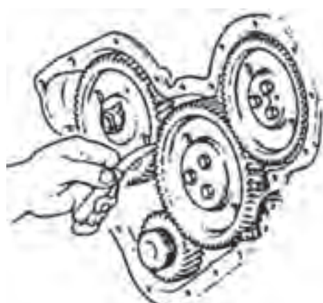
شکل ۷۱-۴ اندازه‌گیری لقی بین چرخ‌دنده‌ها با فیله
