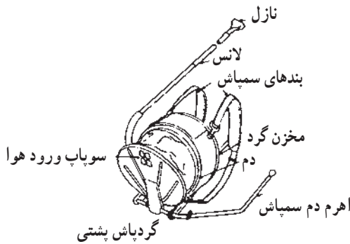
شکل ۳-۱۵- گردپاش های پشتی بی موتور
