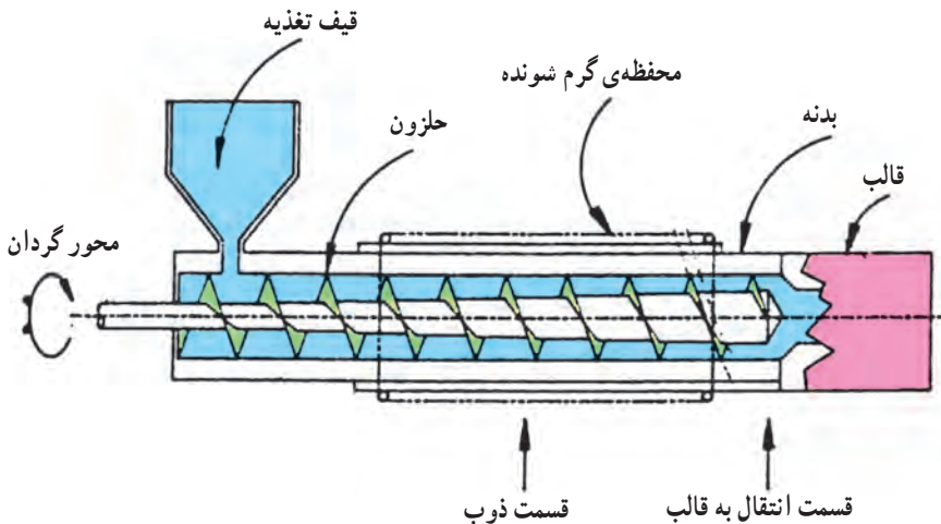
شکل ۱۸-۱- اکسترودر حلزونی مخصوص مواد پلیمری (تزریق پلاستیک)
