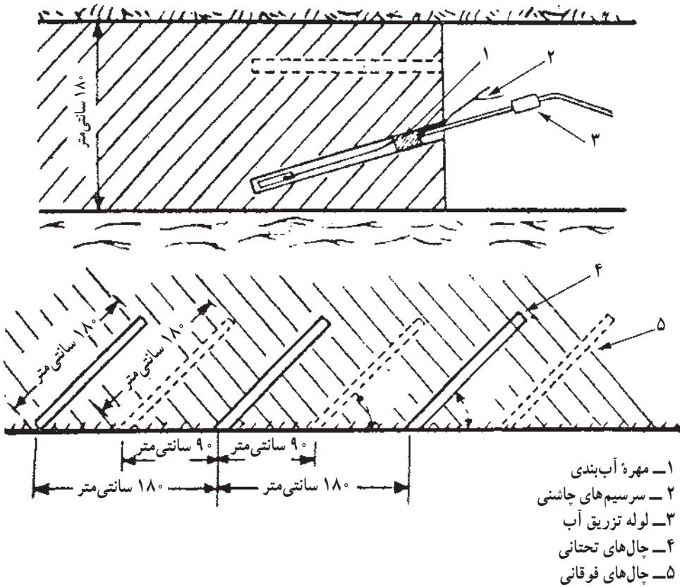
شکل ۳۱-۸- آتش کاری زغال در جا (برش و مقطع عمودی)
