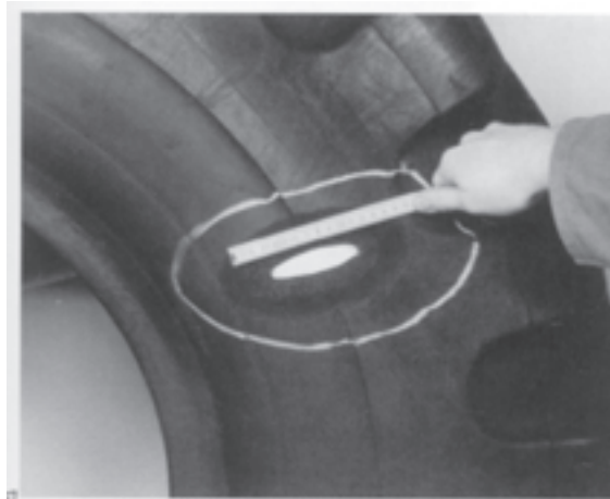
شکل ۵-۱۶-۶-۵ اندازه‌گیری ابعاد حفره
