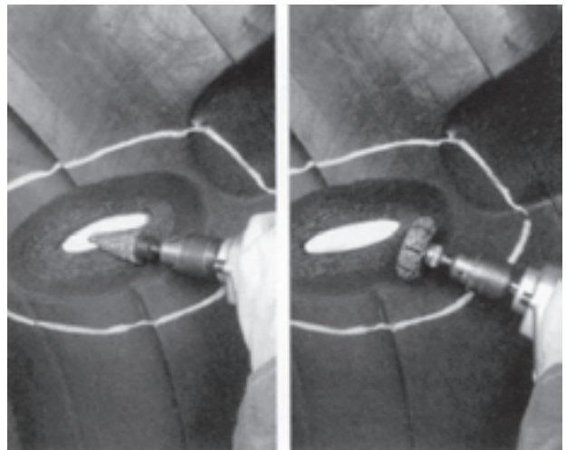
شکل ۳-۱۶-۶-۳ سنگ زدن اطراف حفره
