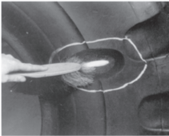
شکل ۴-۱۶-۶-۴ برس زدن اطراف حفره
