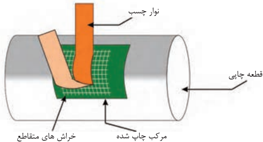
شکل ۴۱-۳ روش تست نوار چسب
