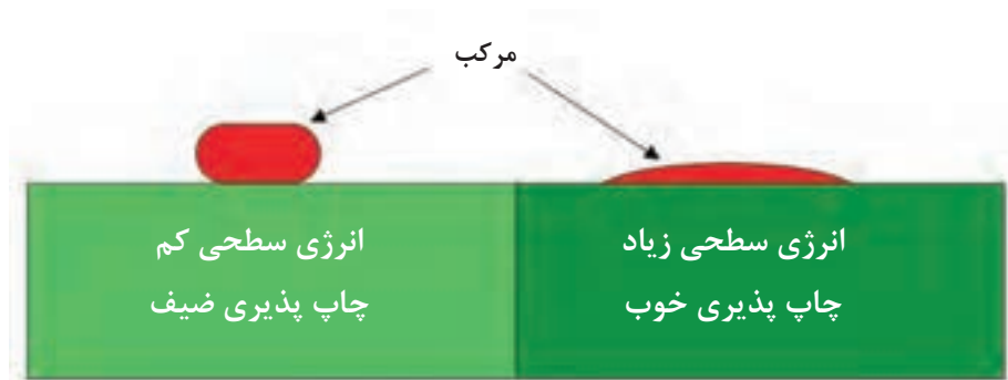
شکل ۳۸-۳ کشش سطحی در چسبندگی در مواد خیس پذیر و خیس ناپذیر
