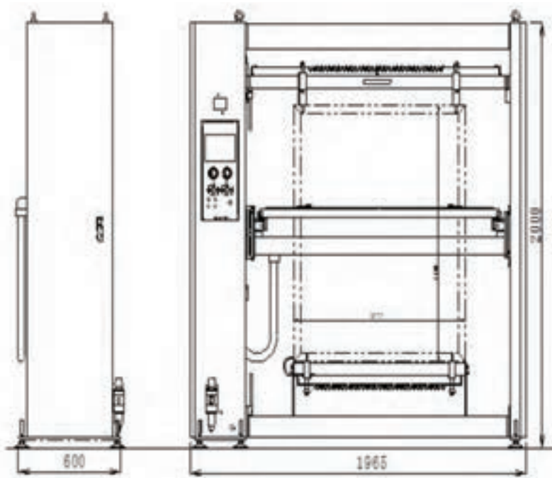
شکل ۱-۱ شمای دستگاه لاک کشی خودکار
