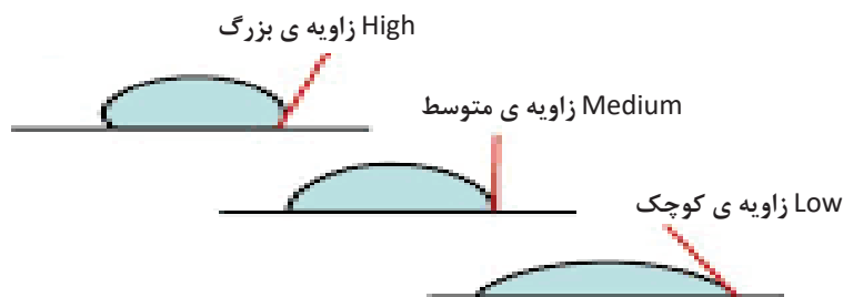
شکل ۵-۲ اندازه گیری کشش سطحی
