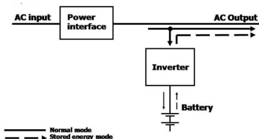
شکل شماره ۳- ساختار تکنولوژی Line-Interactive
