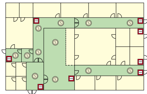
شکل ۷-سیستم نوع L4
