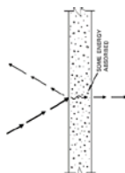
شکل ۲۱- جذب، انعکاس و عبور انرژی صوتی از اجسام
