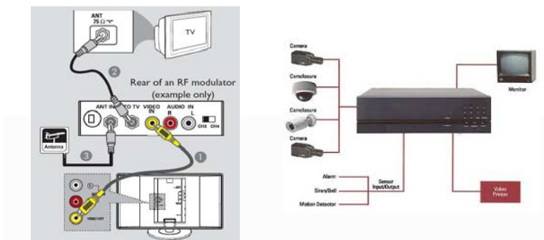
شکل ۹-... اتصال مدلاتور
