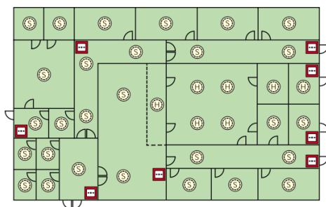
شکل ۱۰-سیستم نوع L1
