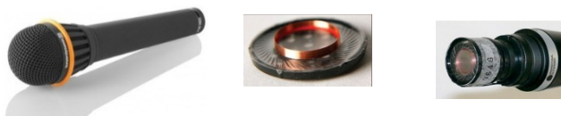
شکل ۳۶- اجزای میکروفن دینامیکی
