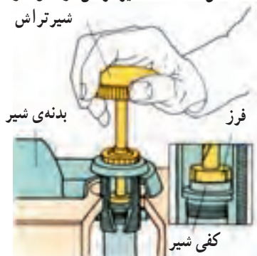
شکل ۲-۶۹- طرز استفاده از شیر تراش
