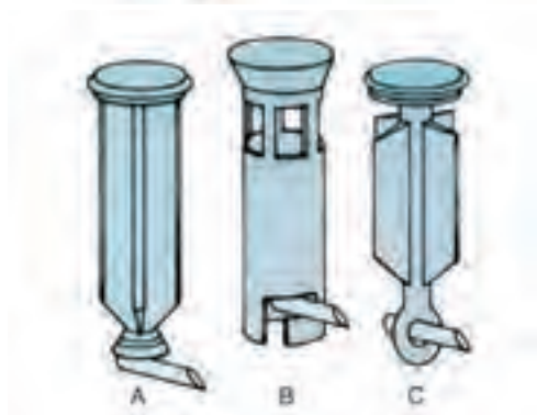
شکل ۴-۲- جزئیات ارتباط ضامن با سرپوش فلزی زیراب
