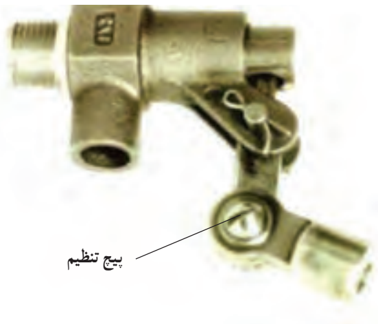
شکل ۲-۱۱۵- بدنه‌ی یک شیر شناور
