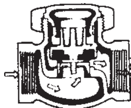
شکل ۲-۱۰۰ - شیر یک طرفه‌ی سوپاپی
