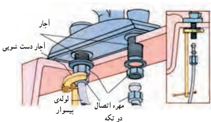
شکل ۱۲۸-۲- ب- نحوه بستن شیلنگ و مهره در شکل نشان داده شده است.
