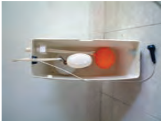
شکل ۳-۲۳۳- مخزن فشاری برش نخورده
