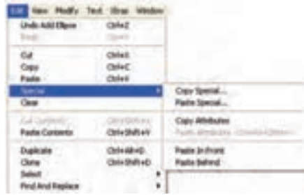
شکل ۵۳-۶ منوی Edit
