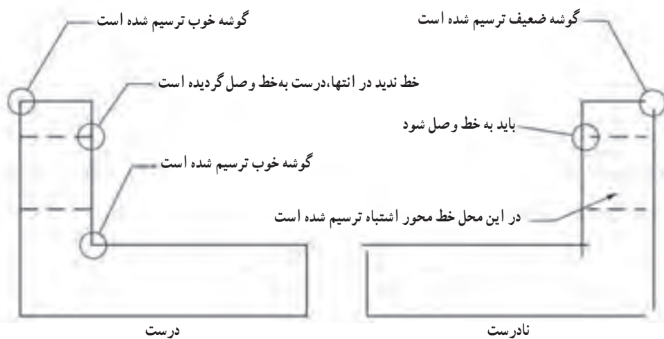
شکل ۲۰-۶- نمونه‌ای از یک نقشه ترسیم شده خوب و ضعیف
