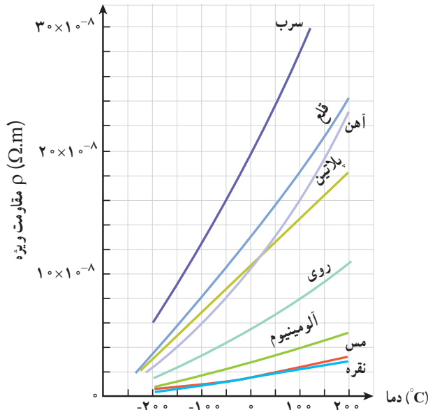
شکل ۸-۳ نمودار تقریبی مقاومت ویژه چند فلز در یک محدوده دمایی
