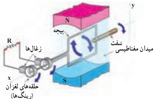
شکل ۱۴-۴ اجزای یک مولد (ژنراتور) ساده ac. حرکت مکانیکی از طریق میل‌گردان، سبب چرخیدن پیچه در میدان مغناطیسی می‌شود و جریانی متناوبی را در مدار به وجود می‌آورد.
