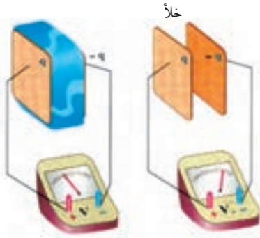
شکل ۱-۲۹ با وارد شدن دی الکتریک در بین صفحه‌های خازن، اختلاف پتانسیل اولیه V_0 به مقدار کوچک‌تر V کاهش یافته است.
