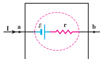
شکل ۲-۱۱ توان خروجی از باتری شکل از رابطه P = (V_b - V_a)I به دست می آید.
