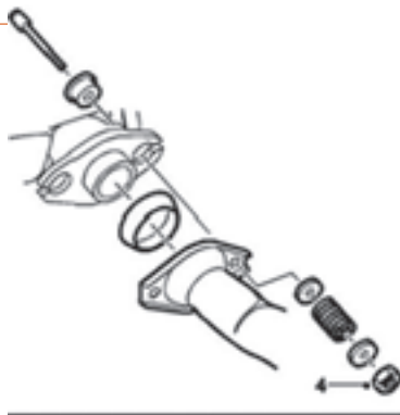
انفجاری گلویی آگزوز شکل ۳-۴۰
