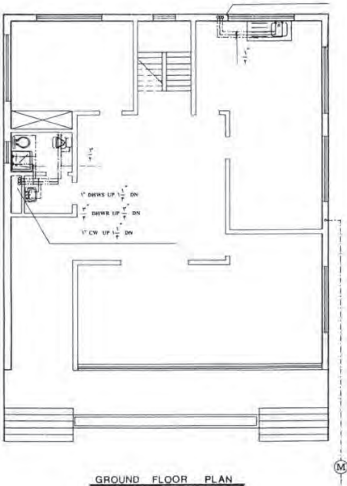
▲ شکل ۲۰-۷- بلان طبقه همکف
