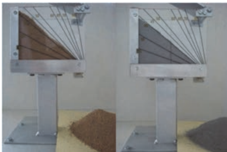
شکل ۳۷- شکل رفتار جریان‌یابی گرانول‌های خشک (سمت چپ) و تر (سمت راست)
