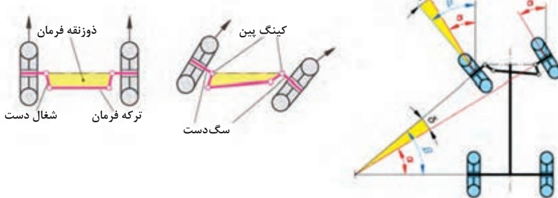
شکل ۱۳- هندسه فرمان
