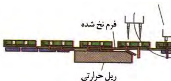
شکل ۱۸- ریل حرارتی و ذوب شدن بست‌های نخ
