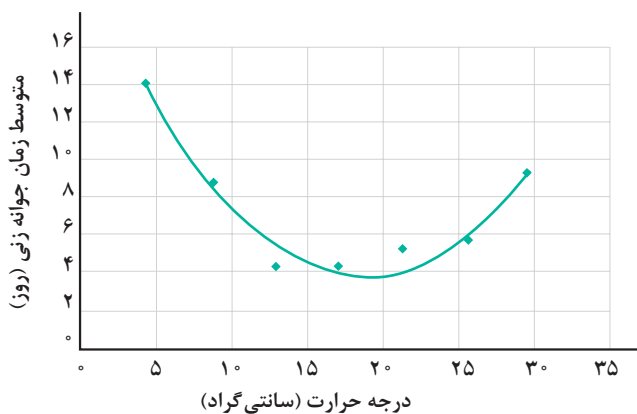
رابطه طول مدت جوانه زنی با میانگین دمای روزانه در یک نوع بذر
