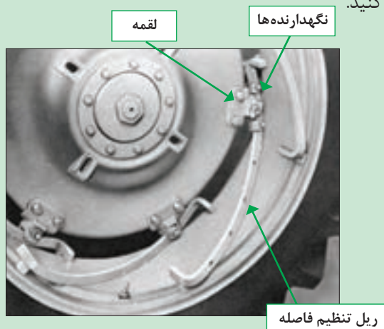
شکل ۳۵-۵- رینگ ریلی
