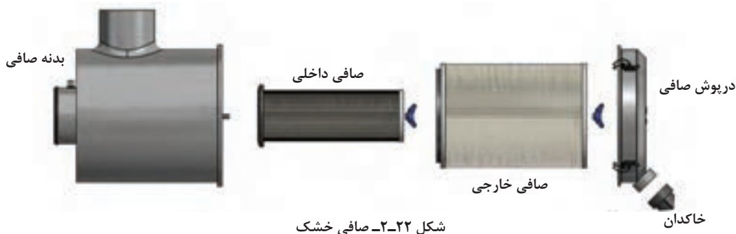
شکل ۲۲-۲- صافی خشک
