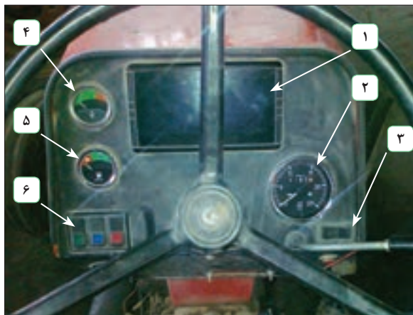
شکل ۳- وسایل اندازه‌گیری و هشداردهنده تراکتور
