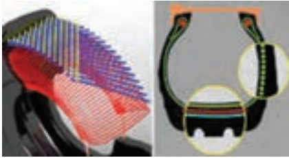
شکل ۵-۱۱- تایر رادیال
