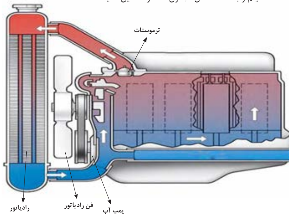
شکل ۲-۳۶- سیستم خنک‌کننده
