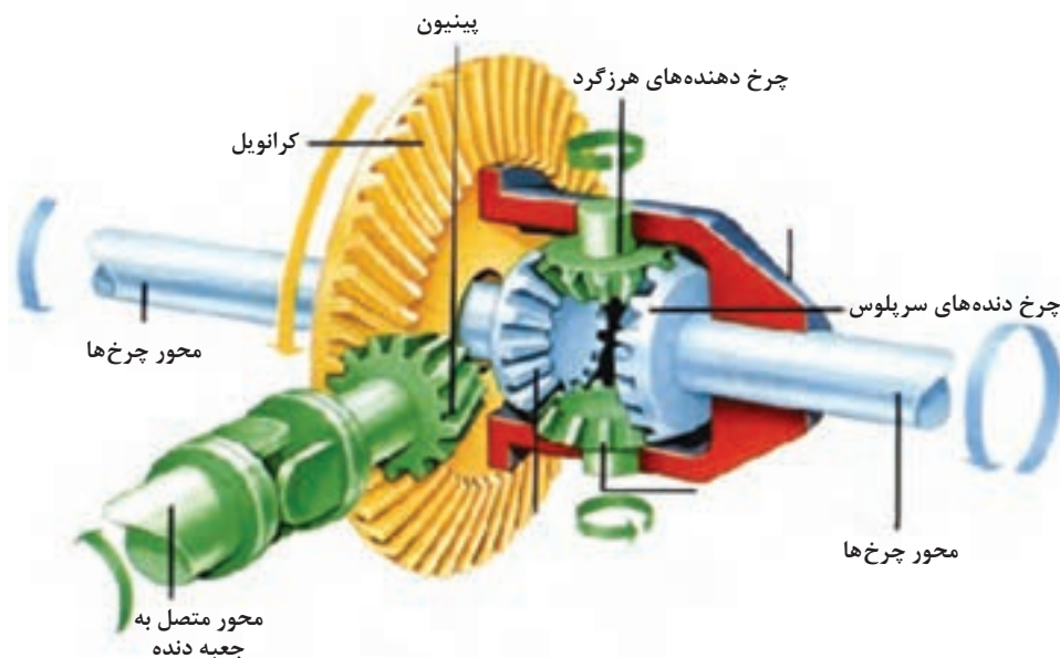
شکل ۲۲-۳- اجزای دیفرانسیل
