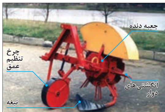
شکل ۸- سیب‌زمینی‌کن دوار
