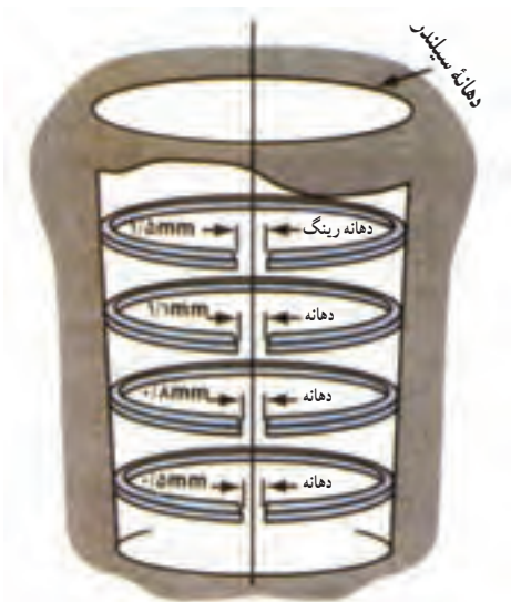
شکل ۱۲۹-۴- اندازه دهانه رینگ در محل‌های مختلف سیلندر
