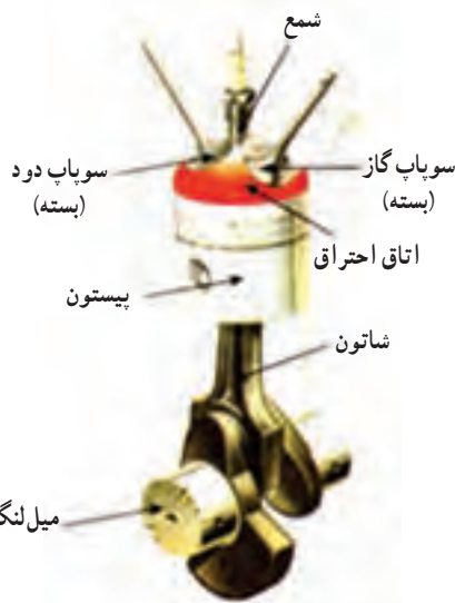
شکل ۴-۱- قطعاتی که در موتور، حرکت رفت و برگشتی را به دورانی تبدیل می‌کنند
