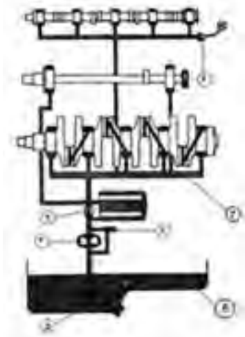
شکل ۱-۷- اجزای مدار روغن کاری
