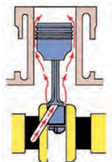
شکل ۴-۷- روغن کاری یاتاقان متحرک و رینگ‌ها
