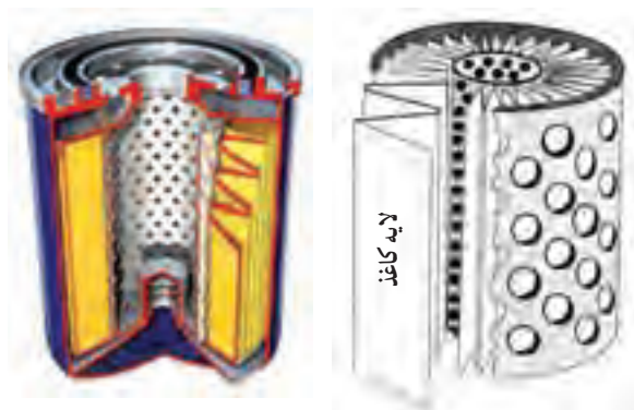
شکل ۱۵-۷- طرز قرار گرفتن لایه کاغذی در صافی
