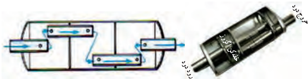
شکل ۲۵-۵- خفه‌کن معکوس
