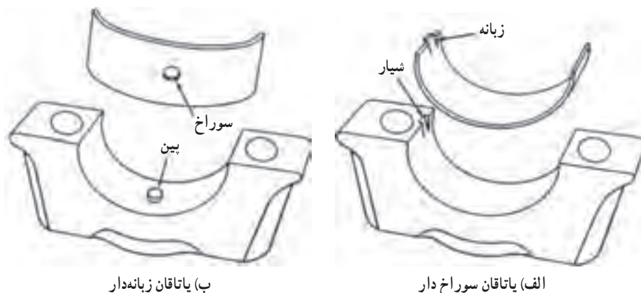
شکل ۴۳-۲- روش‌های جلوگیری از گردش یاتاقان
