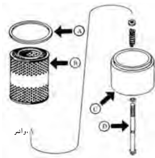
شکل ۵۸-۷ اجزای صافی هیدرولیک
