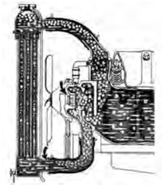
شکل ۳۶-۳- جوش آوردن آب موتور
