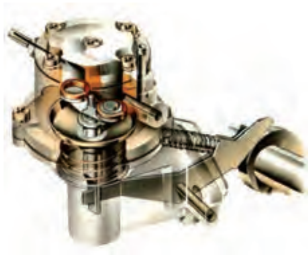
شکل ۷-۴ پمپ مقدماتی دیفراگمی
