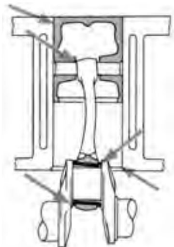
شکل ۱۱۲-۴- محل‌های ساییدگی بر اثر خمیدگی شاتون
