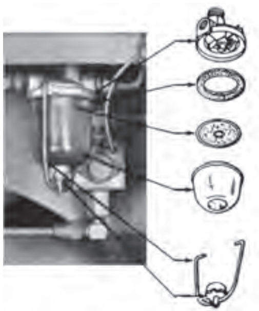
شکل ۱-۴- پیاله رسوبگیر
