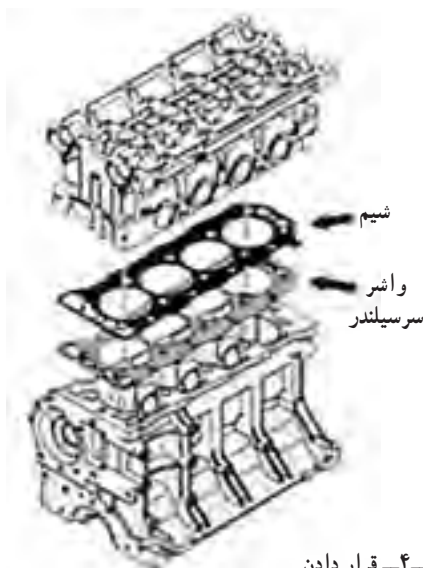
شکل ۳۴-۴- قرار دادن شیم با واشر سرسیلندر
