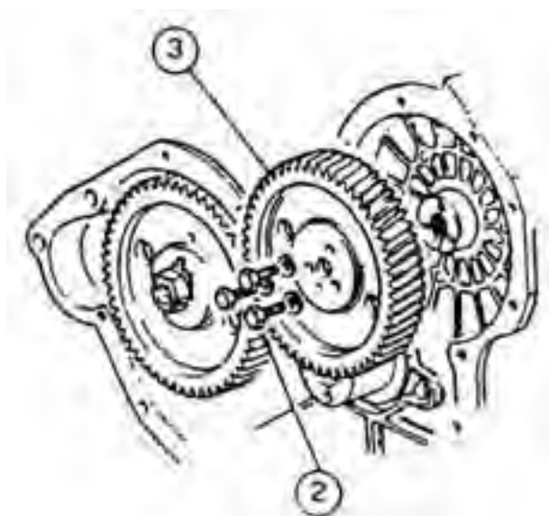
شکل ۷۳-۴- اجزای چرخ دنده پمپ انژکتور
