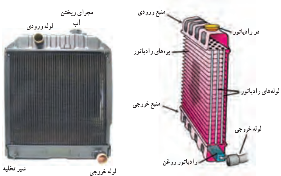
شکل ۳-۳- اجزای رادیاتور
