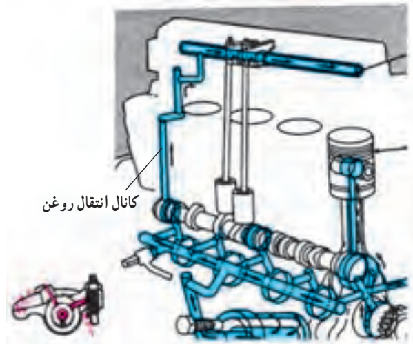
شکل ۷-۷- کانال انتقال روغن به سر سیلندر و محور اسبک
