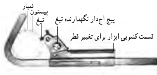
(الف) ابزار تمیزکننده شیپار رینگ‌ها
