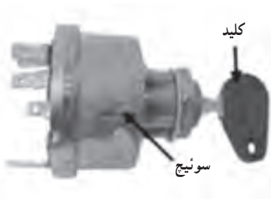
ج) سوئیچ کامل MF285
