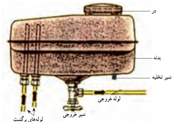
شکل ۲-۴- اجزای باک
