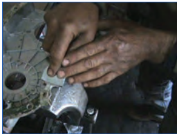
شکل ۴۱-۷- تمیز کردن واشر سینی جلو با کاردک
