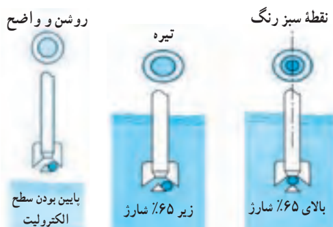
شکل ۳-۶- محل درجه شیشه‌ای در باتری خشک و طرز تعیین شارژ یا دشارژ بودن باتری توسط آن
