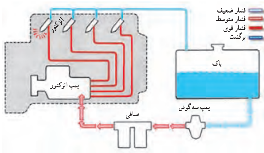
شکل ۳-۴- انواع لوله‌ها در سیستم سوخت‌رسانی دیزل
