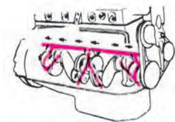
شکل ۳-۷- مسیر روغن از محور ثابت به محور متحرک
