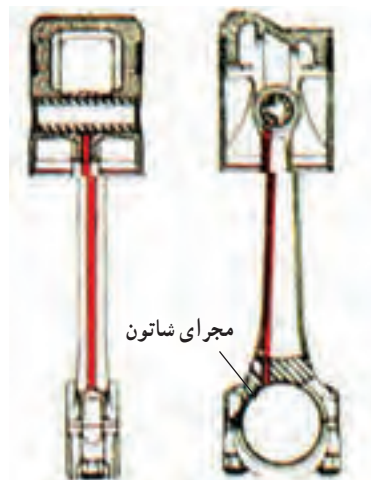
شکل ۵-۷- کانال روغن در شاتون
