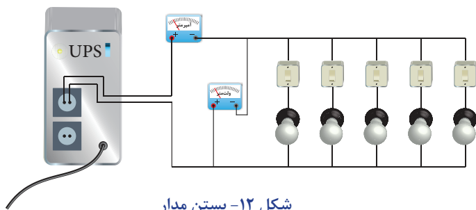
شکل ۱۲- بستن مدار
